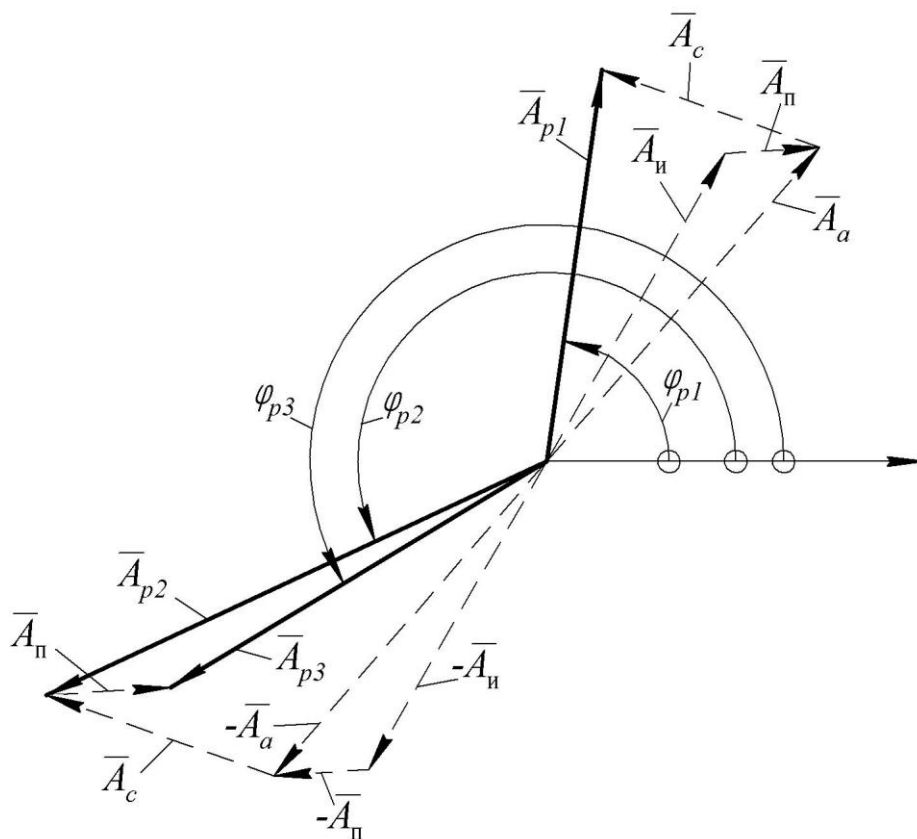
Рис. 4. К определению \bar{A}_e для привода, не допускающего при пуске случайного конечного поворота ротора.
